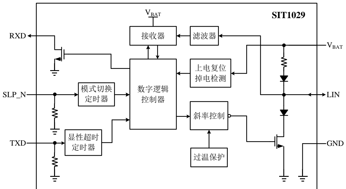
图 3 SIT1029 内部框图
