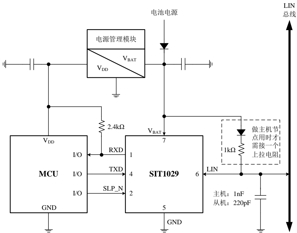
图 7 SIT1029 典型应用示意图
