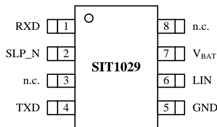
图 2 SIT1029 引脚分布图
